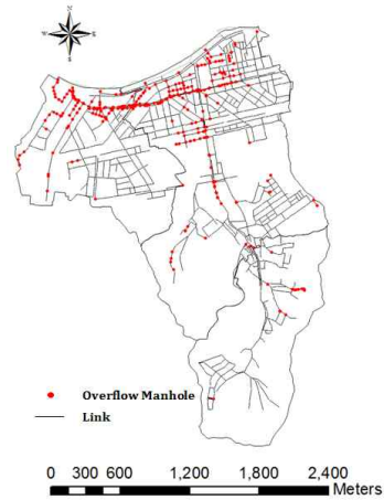
Fig. 9. Overflow Manhole
